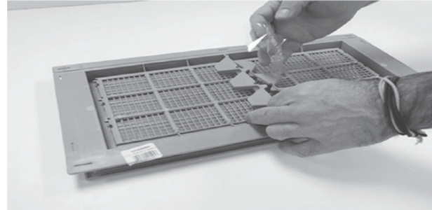
Entfernen Sie die an der Rückseite des Lüfters angebrachten Halterungen. Hinweis: Die Halterungen sind mit links und rechts markiert.
